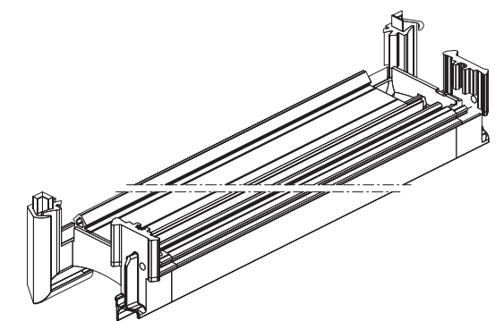
Nové zavírání dveří s izolací polodrážky a vulkanizovanými rohy pro falcové křídlo
