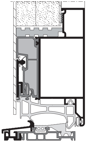
2dílný práh po obvodu s falcovým křídlem
