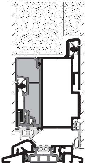
Sešroubovaný práh se zapuštěným křídlem
