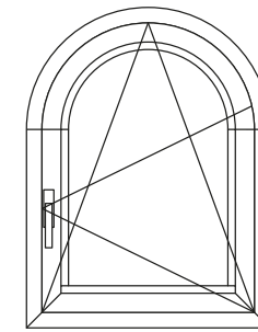
Een draai-kiepraam, naar rechts openend
