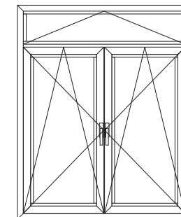
Een kiepvleugel en twee draaiende kiepvleugels
