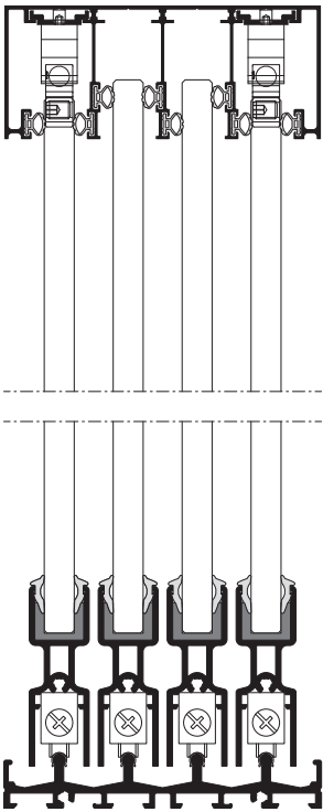
heroal S 20 C, vue en coupe
