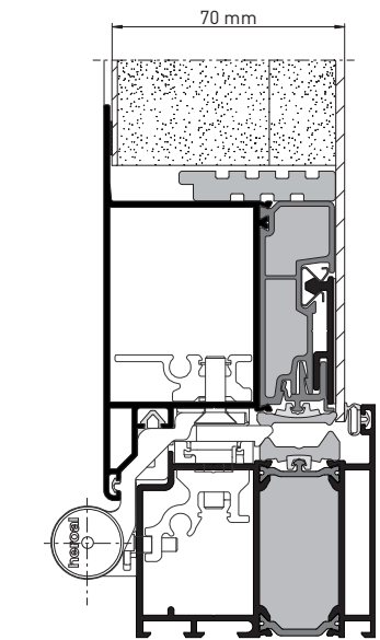
heroal D 72 PF EM 70 mm, Schnittdarstellungen
