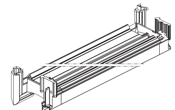
Neue Türabschlusssichtung mit eckvulkanisierter Formecke für Flügel aufschlagend
